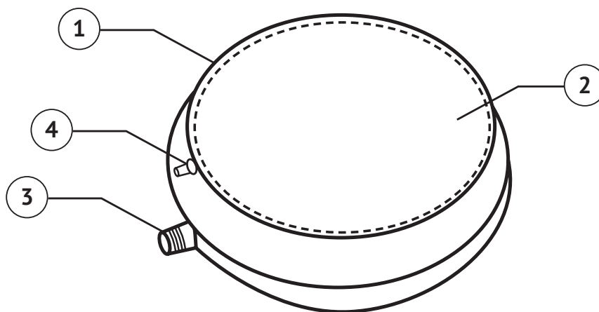
Рисунок 1 – Устройство расширительного бака
