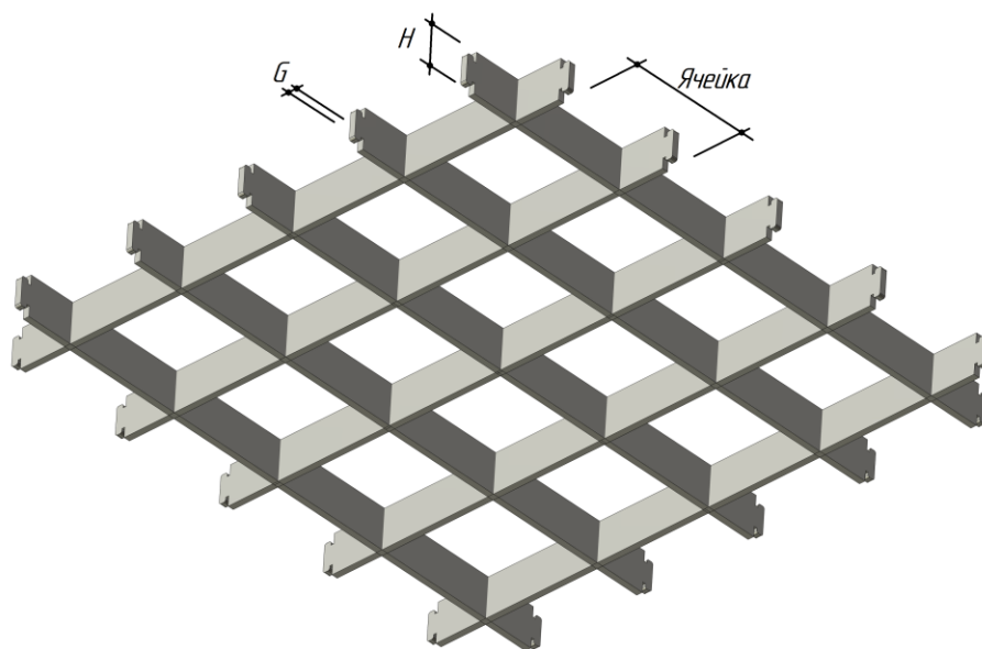
Рисунок 1 – Основные параметры потолка типа «грильято»
