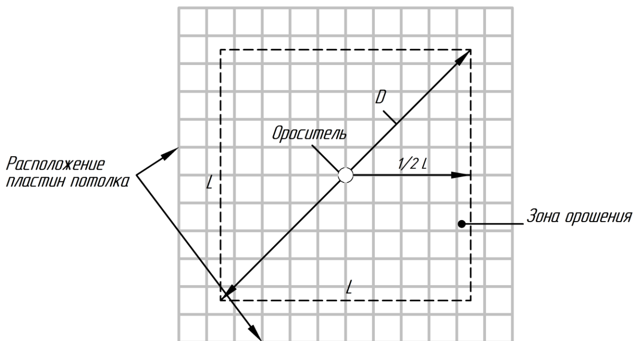
Рисунок 2 – Карта орошения оросителя (распылителя), установленного над подвесным потолком «грильято»
